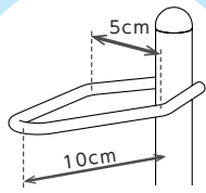
落下防止リング (内寸)
