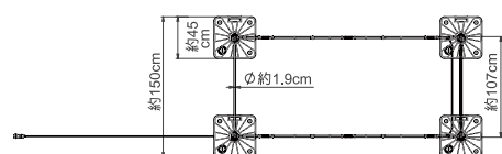
ミストアーチ ジュニア ミスト部：ノズル (シングル3個、ダブル6個)、 ホース内径(φ4mm)、 ホース外径(φ9mm)、 ミスト間隔(0.9m)
